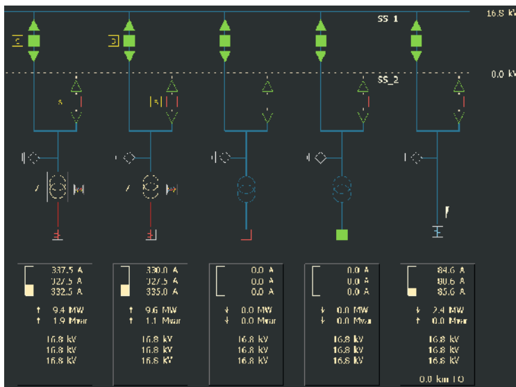
Online-Darstellung einer Mittelspannungsschaltanlage im Leitsystem
